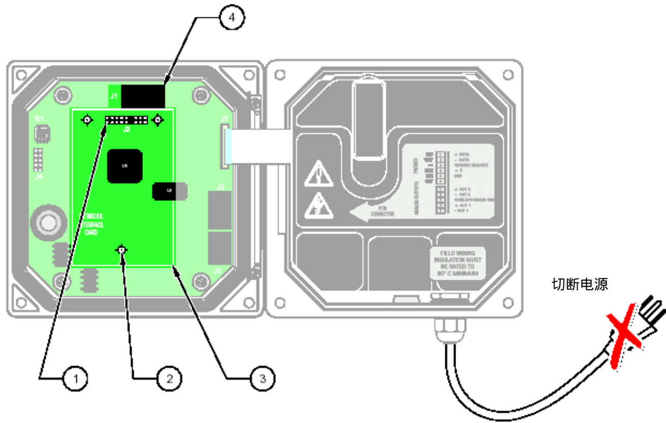
图 22 网络卡在控制器内的位置
